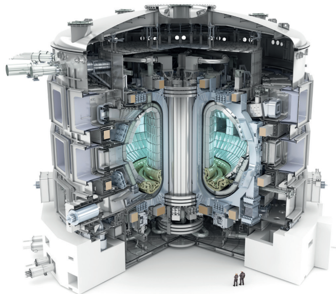
Die Fusionssteanlage ITER wird derzeit in Südfrankreich gebaut. (Grafik: Fusion for Energy)
